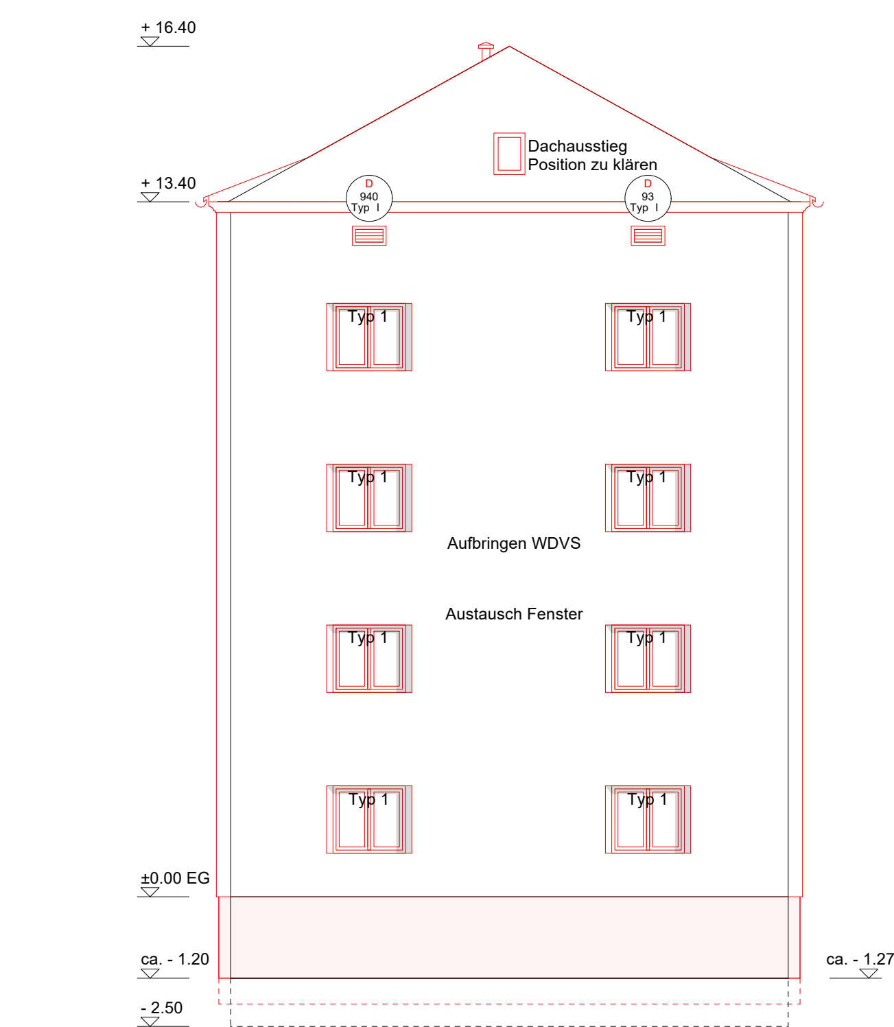
Ostansicht
